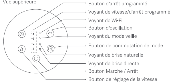
Vue supérieure
