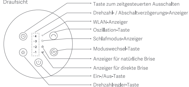
Draufsicht
